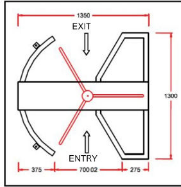
NON - STANDARD TURNSTILE
