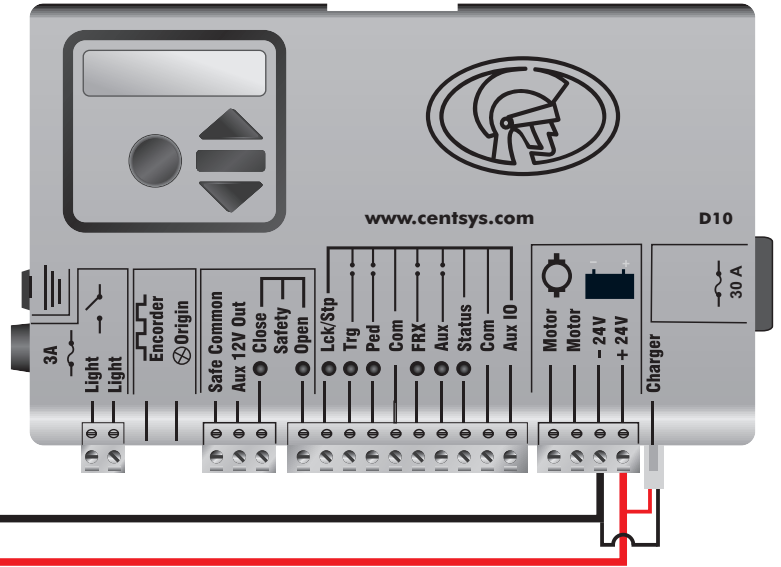
D5 Controller
